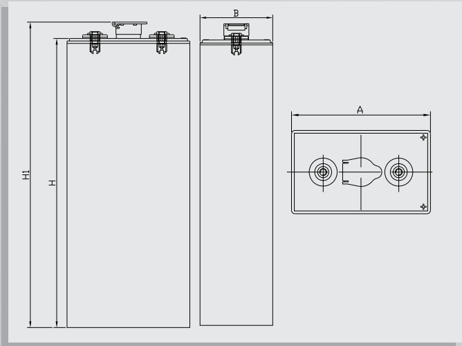
Размеры согласно стандарту IEC 254-2 Std и DIN/EN 60254-2 Std Высота ячеек: погрешность ±3мм
